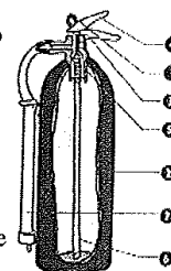
1. Seguro 2. Cuerpo 3. Asa 4. Válvula de resaca 5. Sello 6. Etiqueta 7. Manguera
