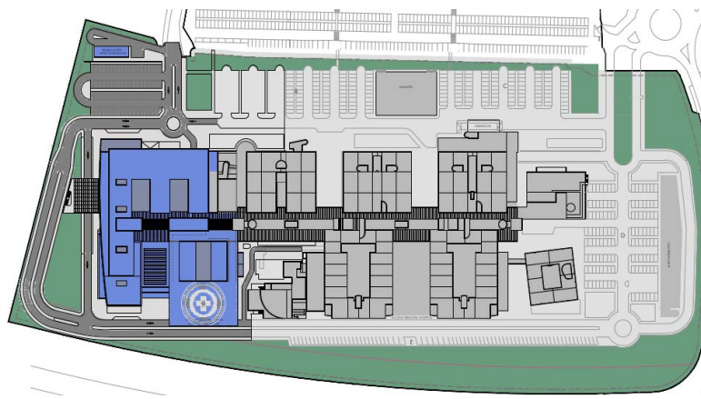
PROYECTO DEL NUEVO HOSPITAL MATERNO INFANTIL. IMPLANTACIÓN MODIFICADO DE ESTUDIO DE DETALLE DE PARCELA DEL HOSPITAL JUAN RAMÓN JIMÉNEZ. HUELVA
